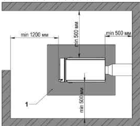
Рис. 5 Установка котла
