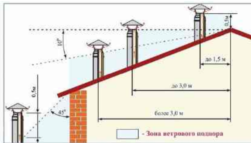
Рис. 9 Высота дымохода.
