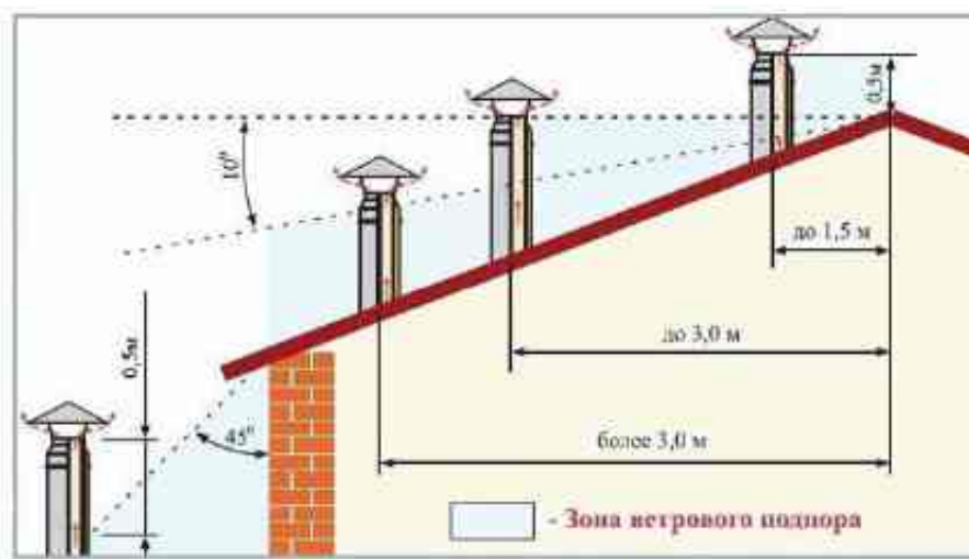
Рис. 7 Высота дымохода.
