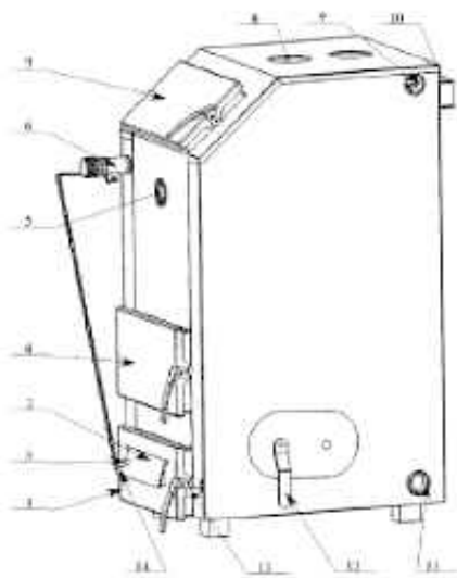
Рис. 1 Схема устройства котла «Магnum» 15/20 кВт
